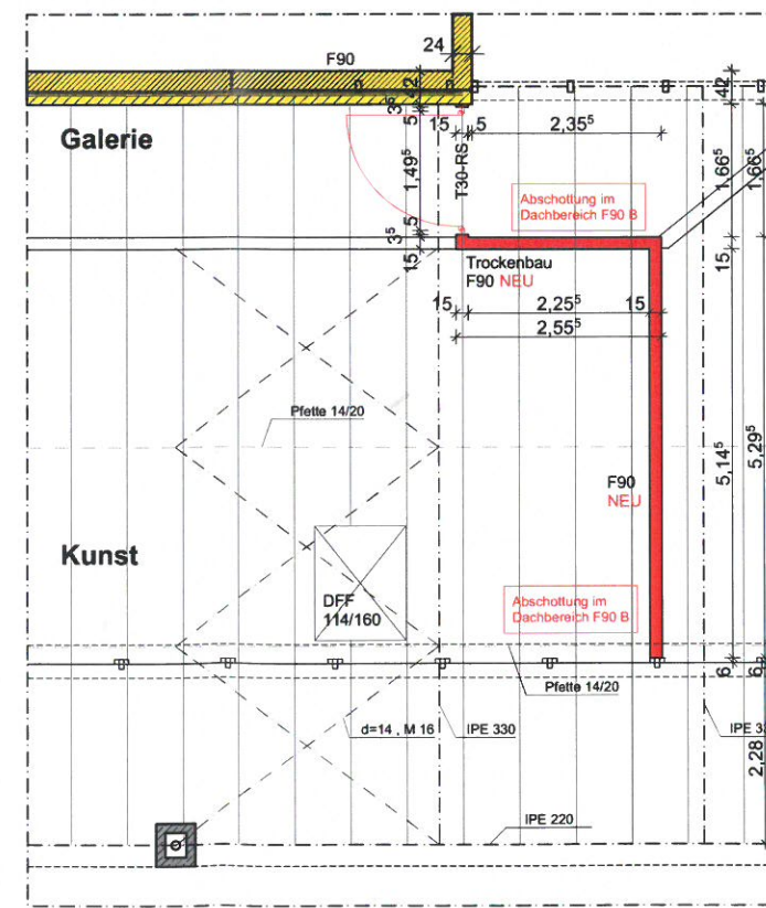
Obergeschoss
