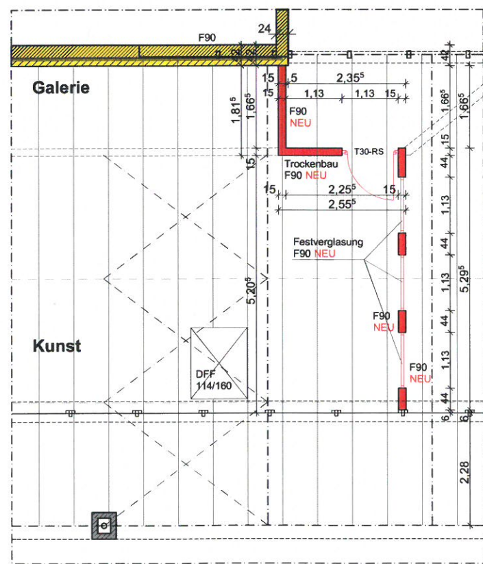
Erdgeschoss
